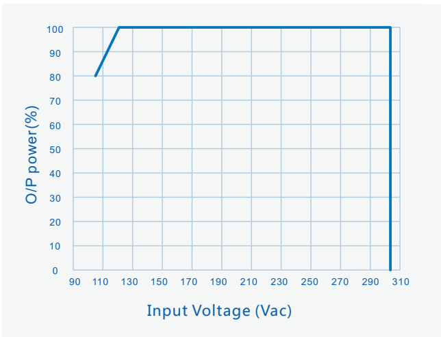
输出功率Vs.输入电压(环温最大55℃)
